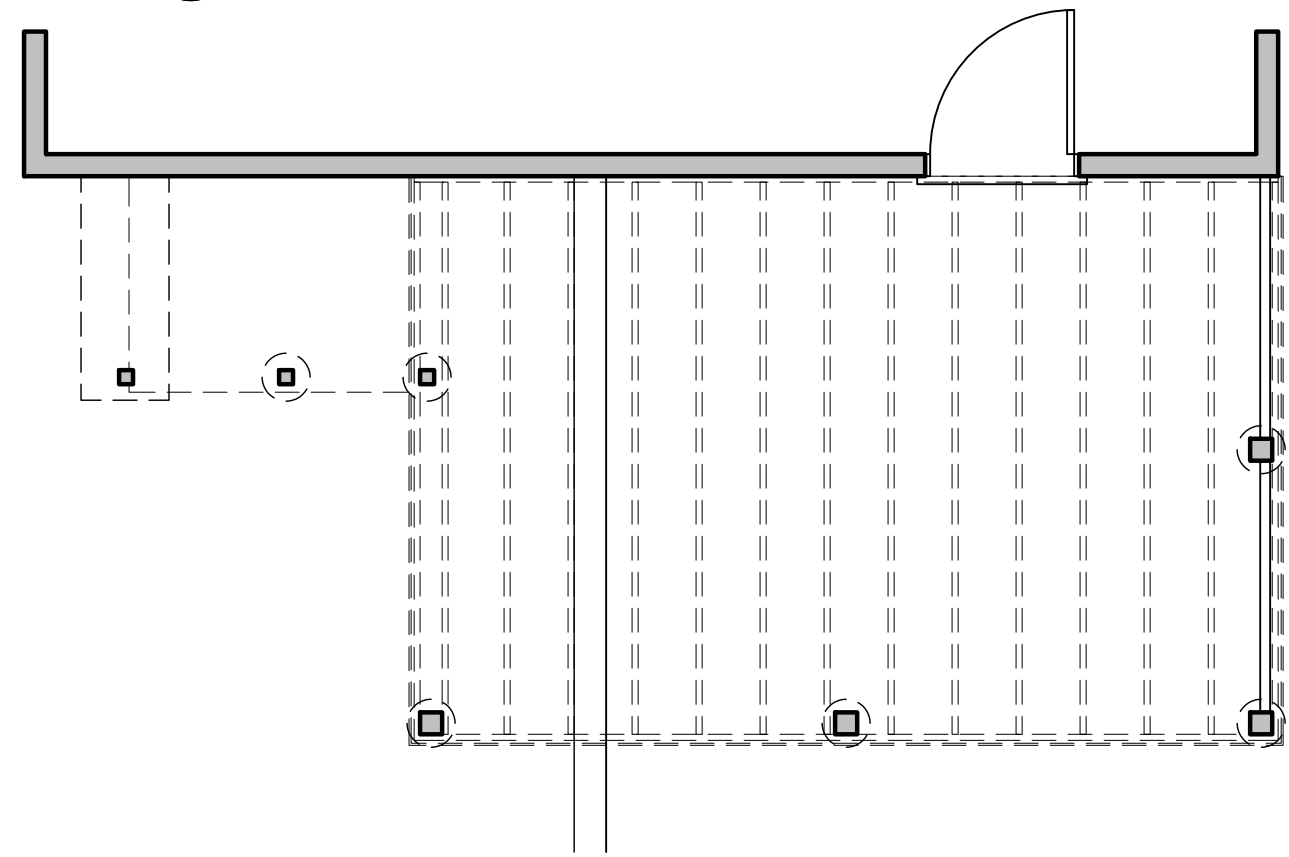
0 PATIO PLAN 1/4"=1'-0"
